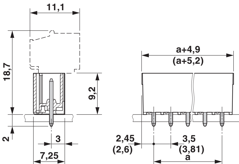
Rysunek wymiarowy
