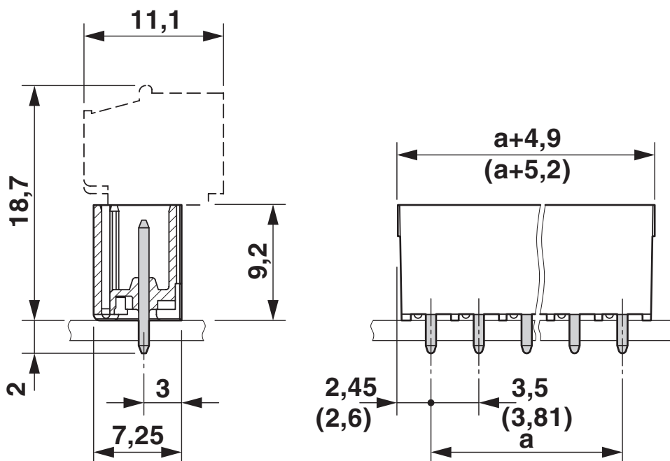
Rysunek wymiarowy
