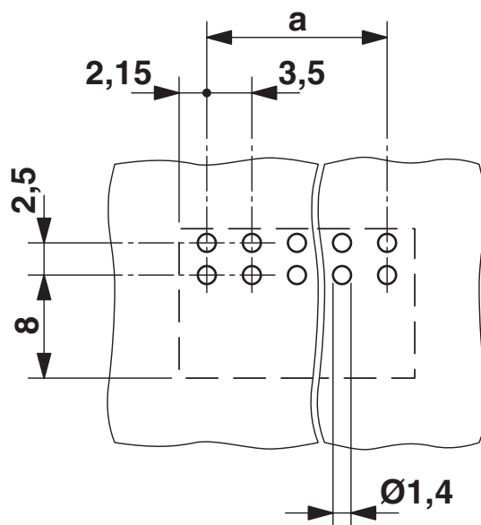
Rysunek wymiarowy
