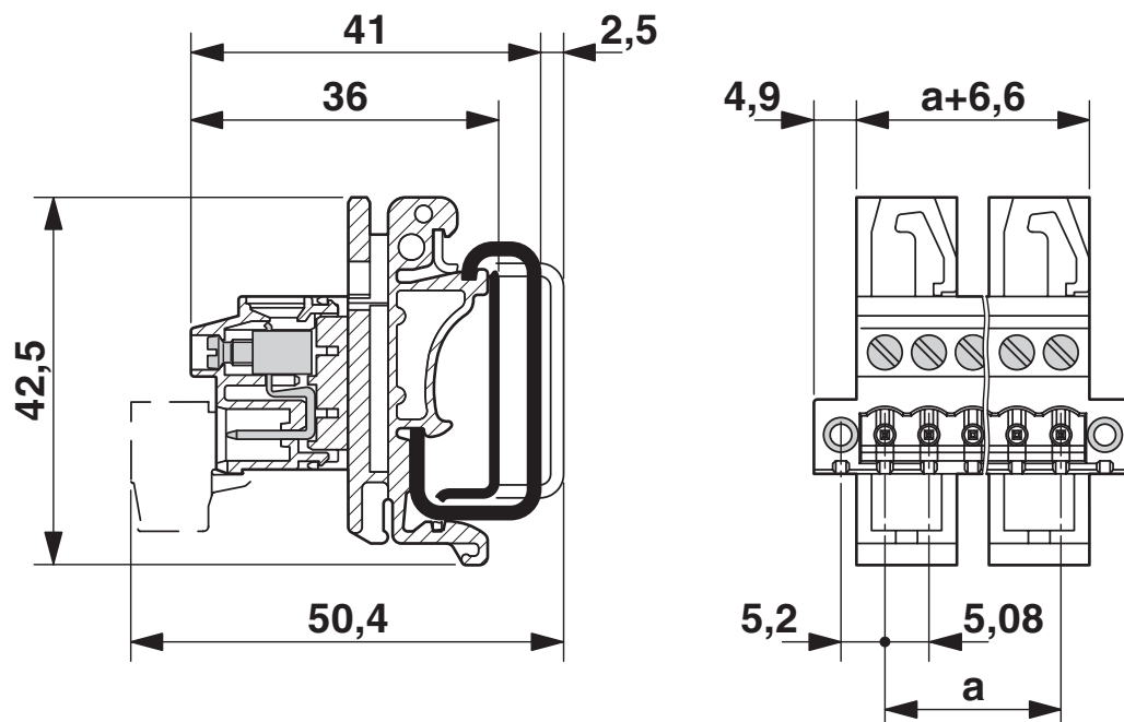
Rysunek wymiarowy
