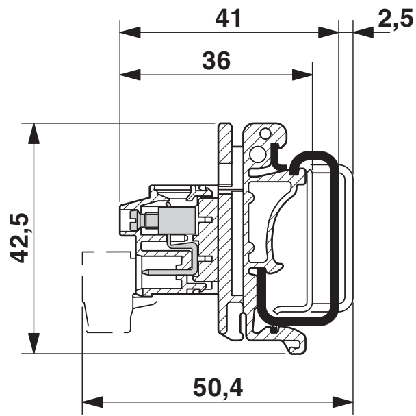
Rysunek wymiarowy
