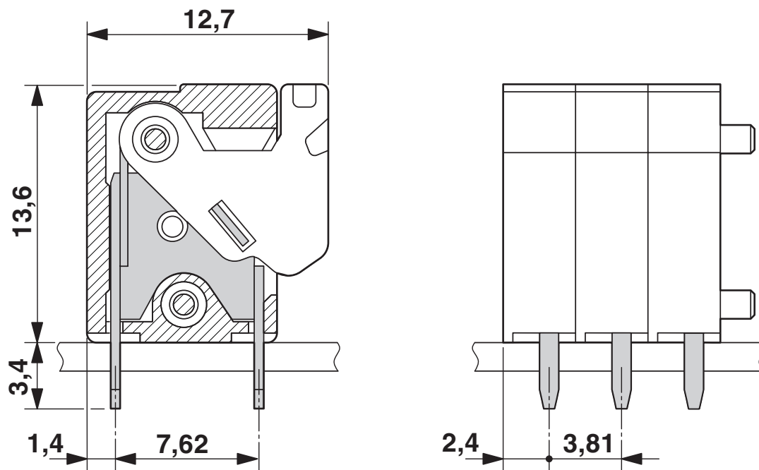
Rysunek wymiarowy
