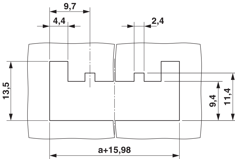
Rysunek schematyczny
