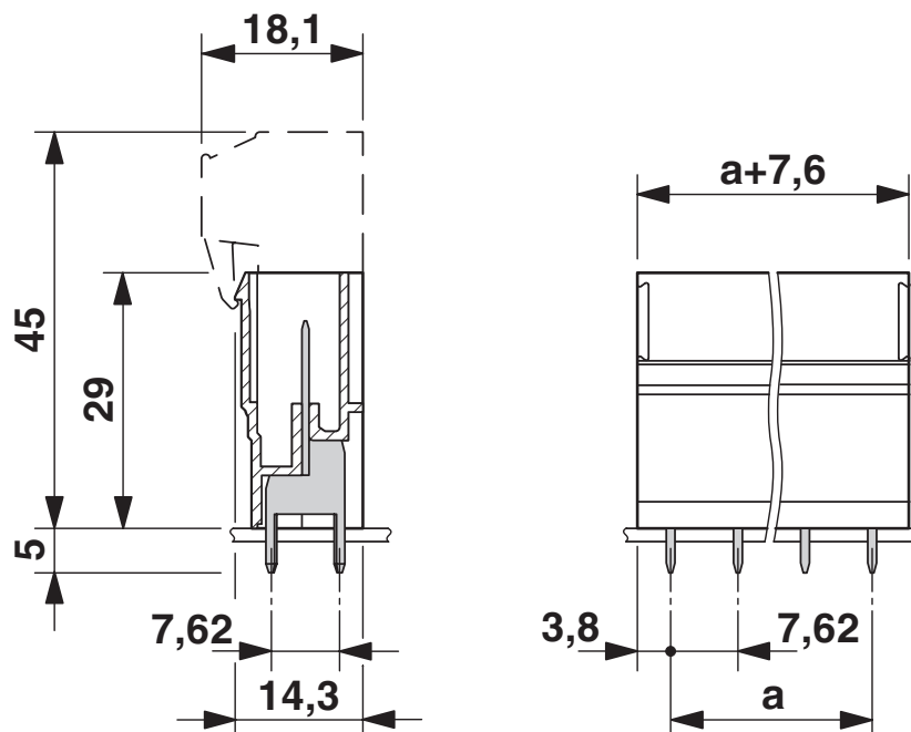
Rysunek wymiarowy
