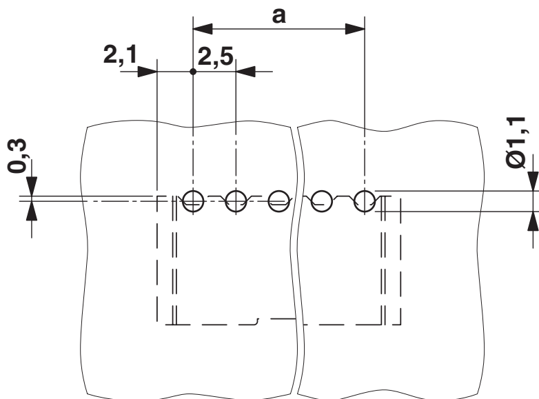
Rysunek wymiarowy
