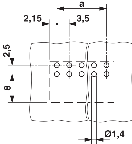
Rysunek wymiarowy
