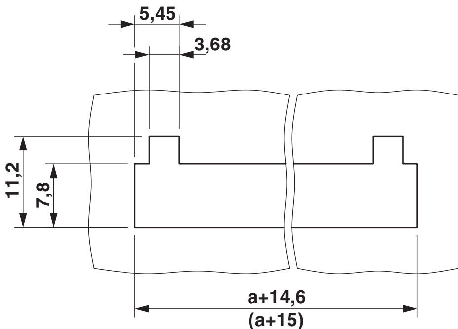
Rysunek wymiarowy
