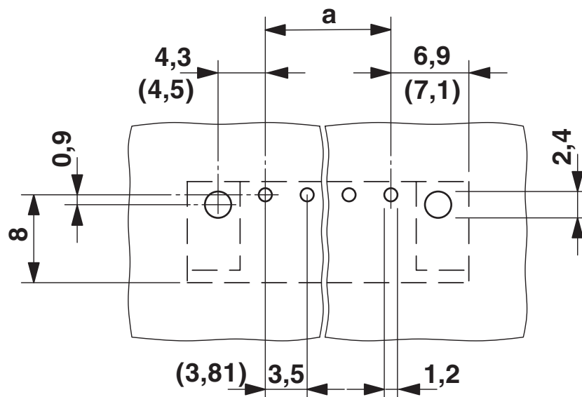
Otworowanie/geometria płytek lutowicznych
