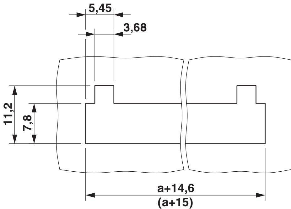
Rysunek wymiarowy
