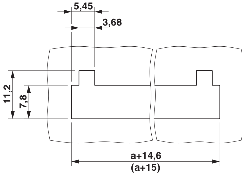
Rysunek wymiarowy
