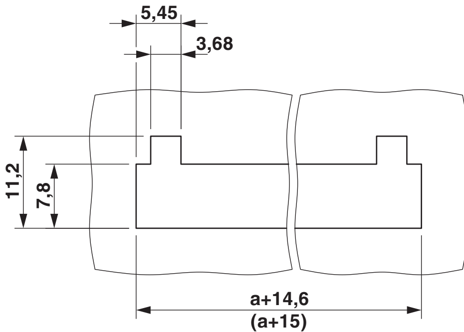
Rysunek wymiarowy
