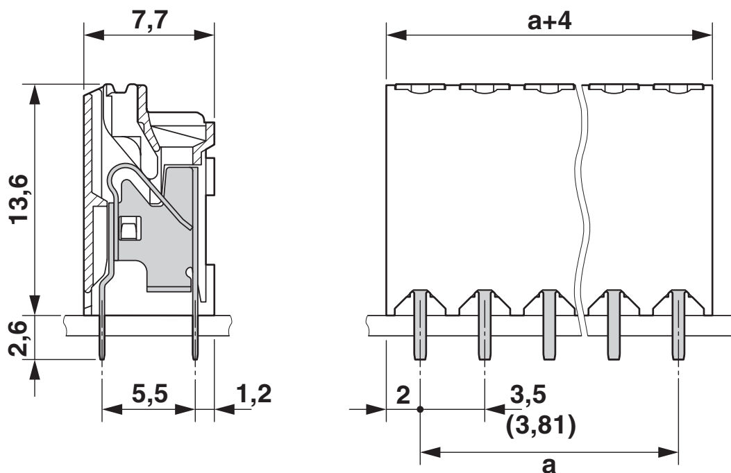
Rysunek wymiarowy
