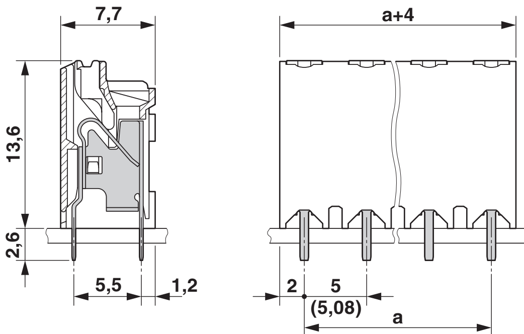
Rysunek wymiarowy
