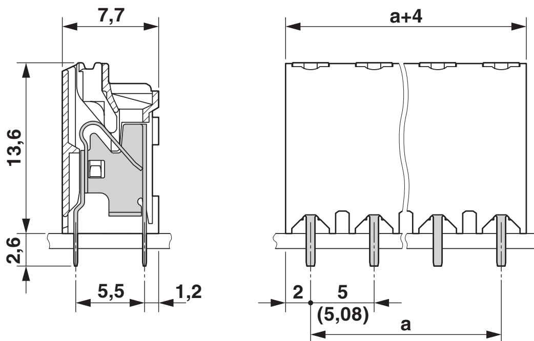
Rysunek wymiarowy
