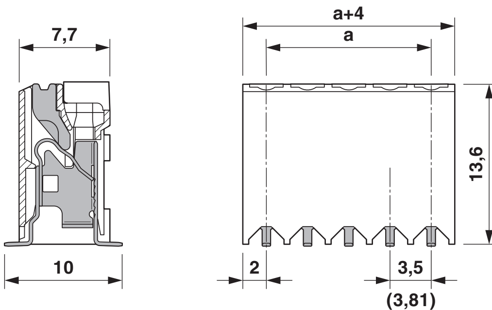
Rysunek wymiarowy
