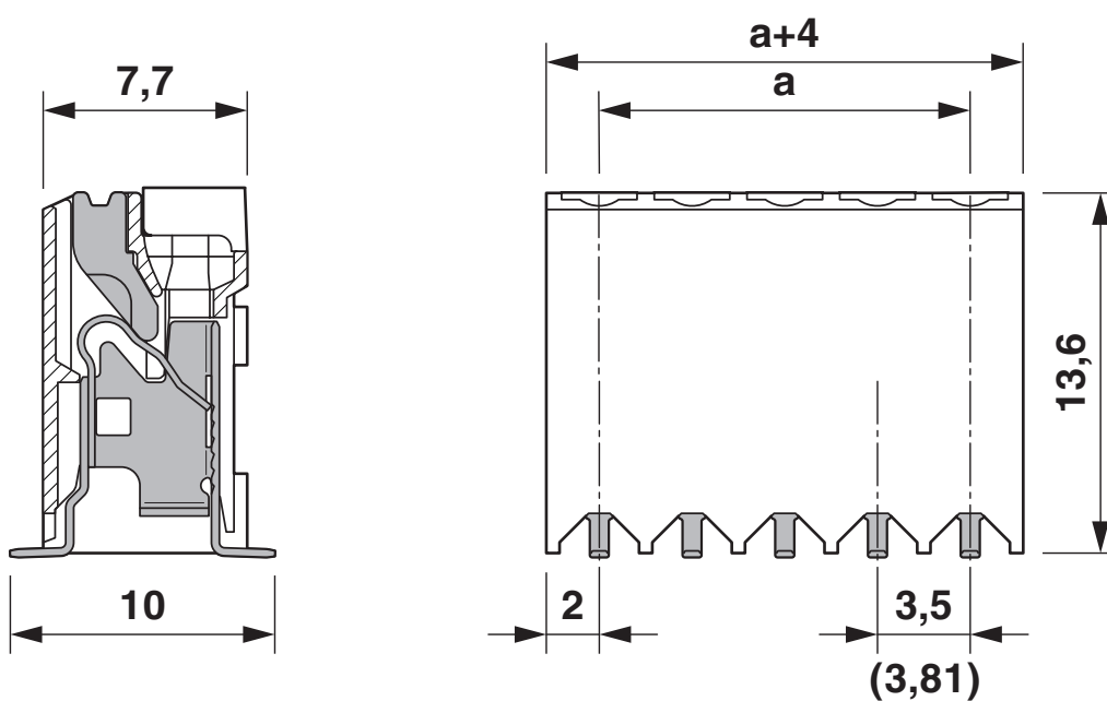
Rysunek wymiarowy
