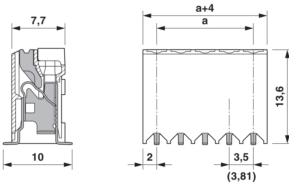
Rysunek wymiarowy
