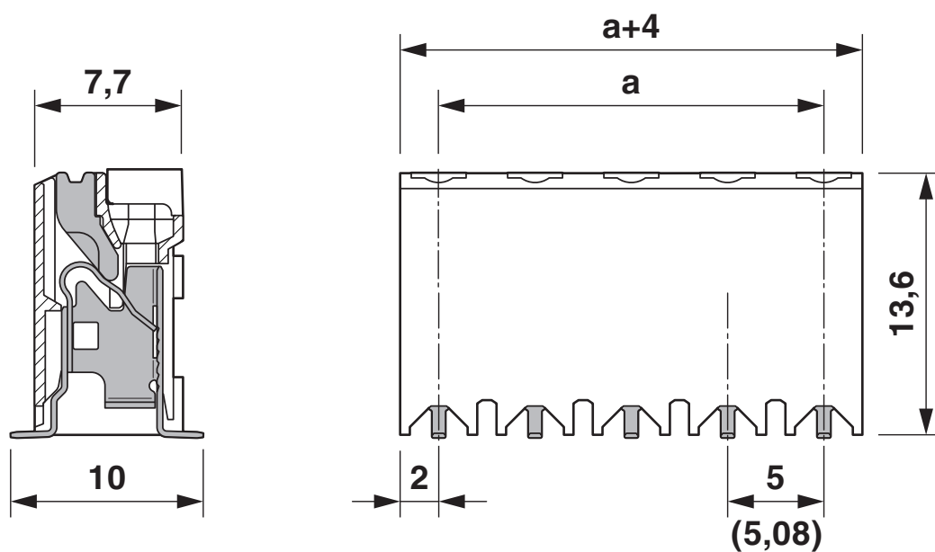
Rysunek wymiarowy
