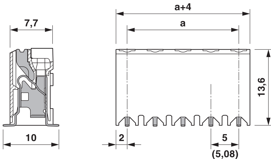
Rysunek wymiarowy
