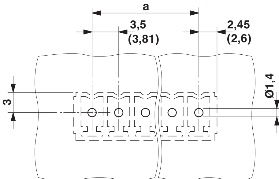
Otworowanie/geometria płytek lutowicznych
