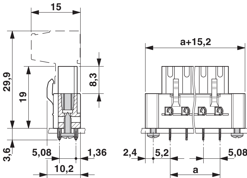
Rysunek wymiarowy
