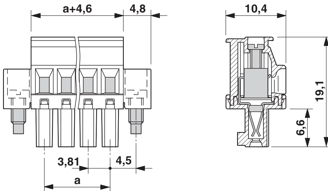
Rysunek wymiarowy
