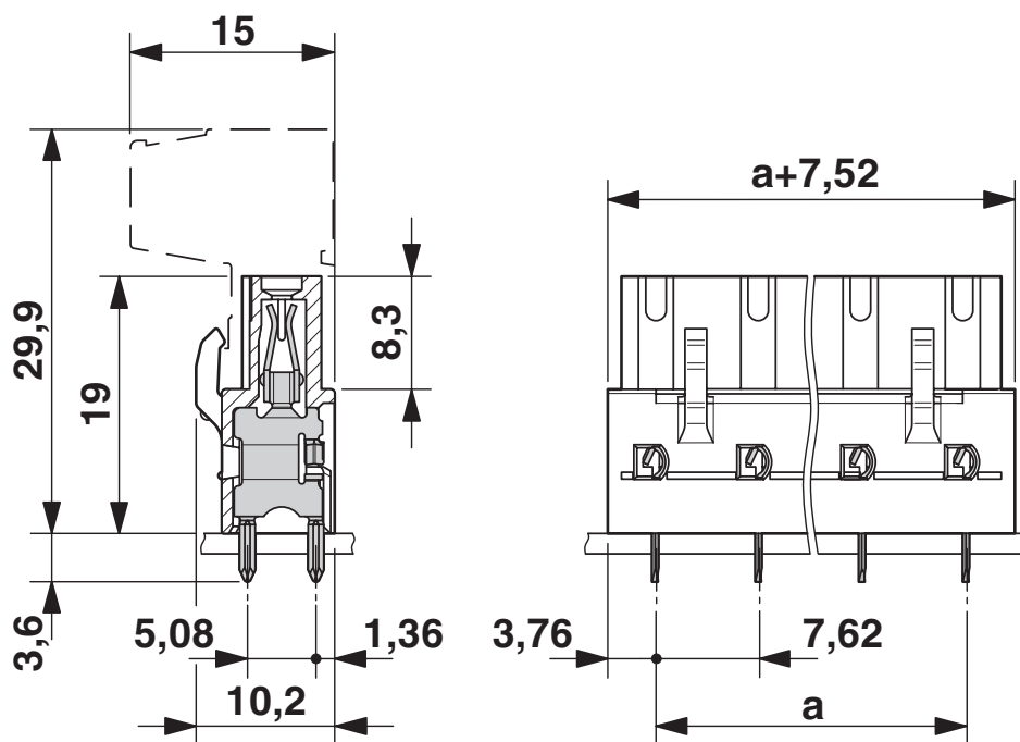
Rysunek wymiarowy
