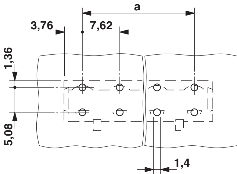
Rysunek wymiarowy
