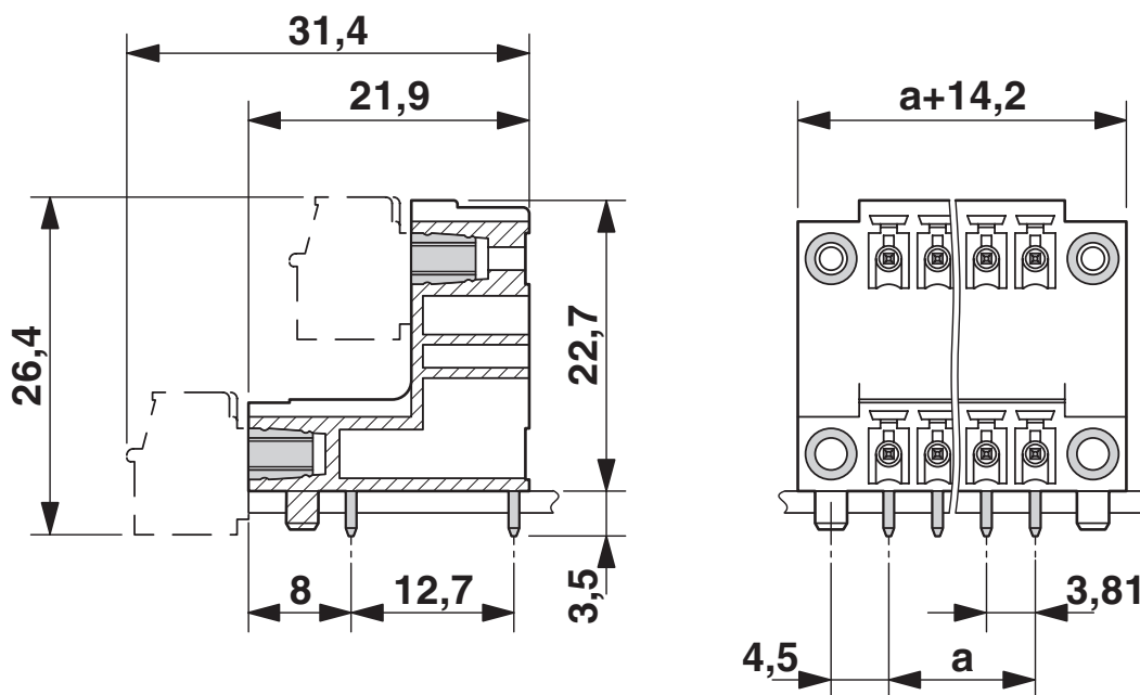
Rysunek wymiarowy
