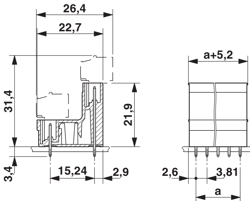
Rysunek wymiarowy
