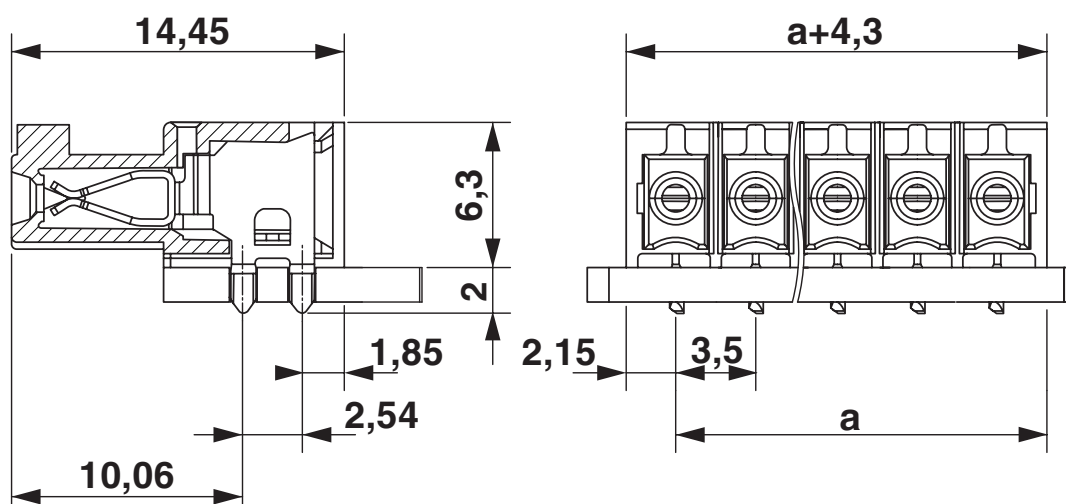
Rysunek wymiarowy
