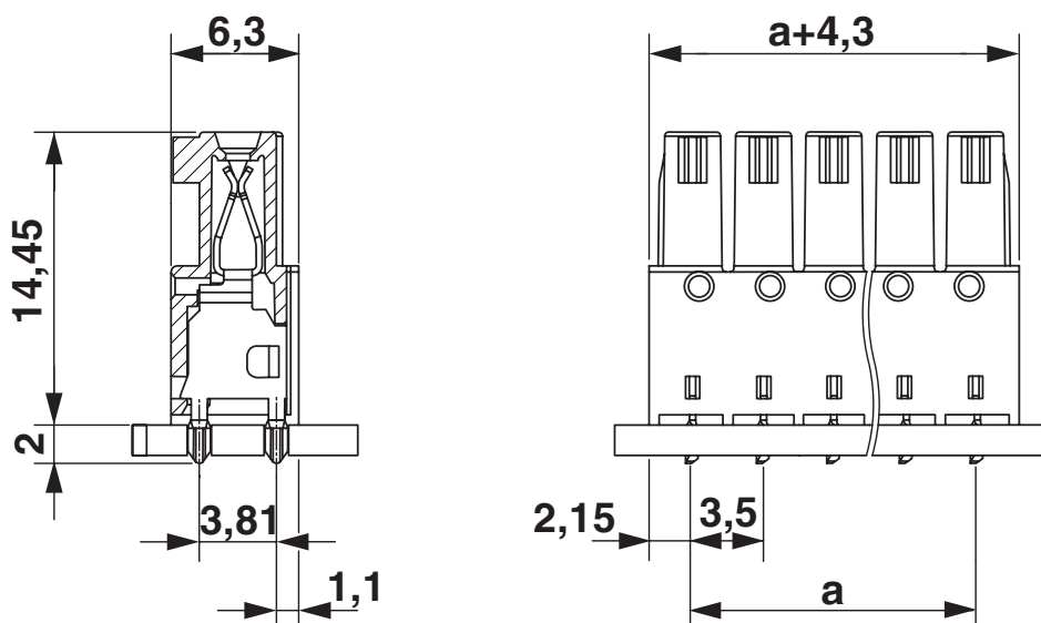
Rysunek wymiarowy
