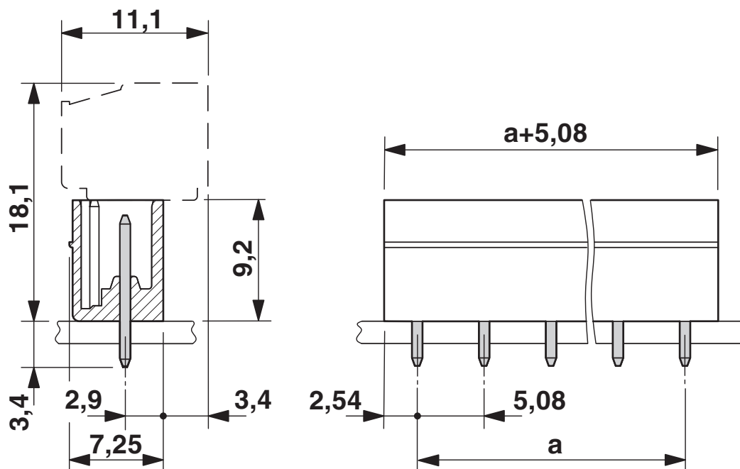
Rysunek wymiarowy
