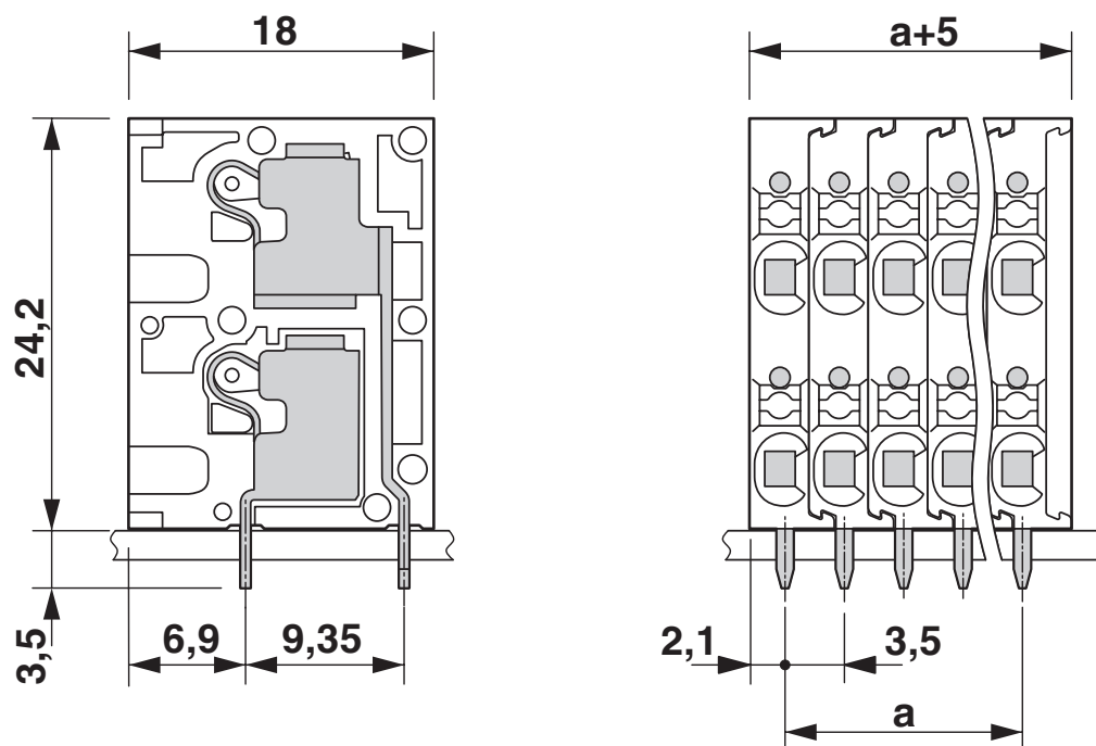
Rysunek wymiarowy
