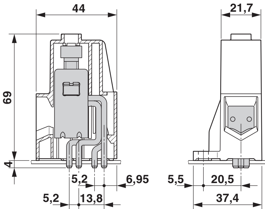
Rysunek wymiarowy
