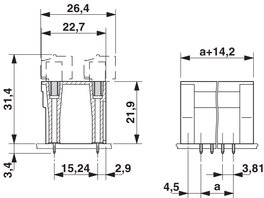
Rysunek wymiarowy
