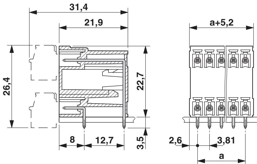
Rysunek wymiarowy
