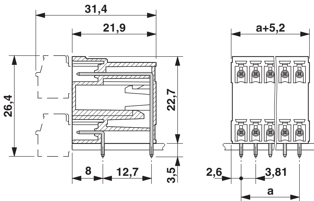
Rysunek wymiarowy
