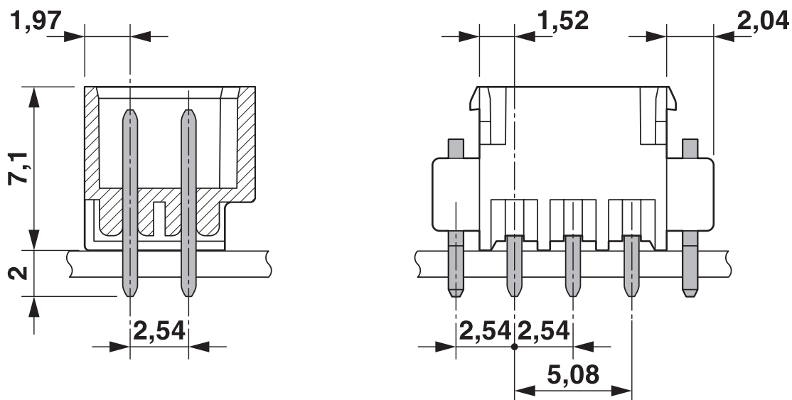
Rysunek wymiarowy
