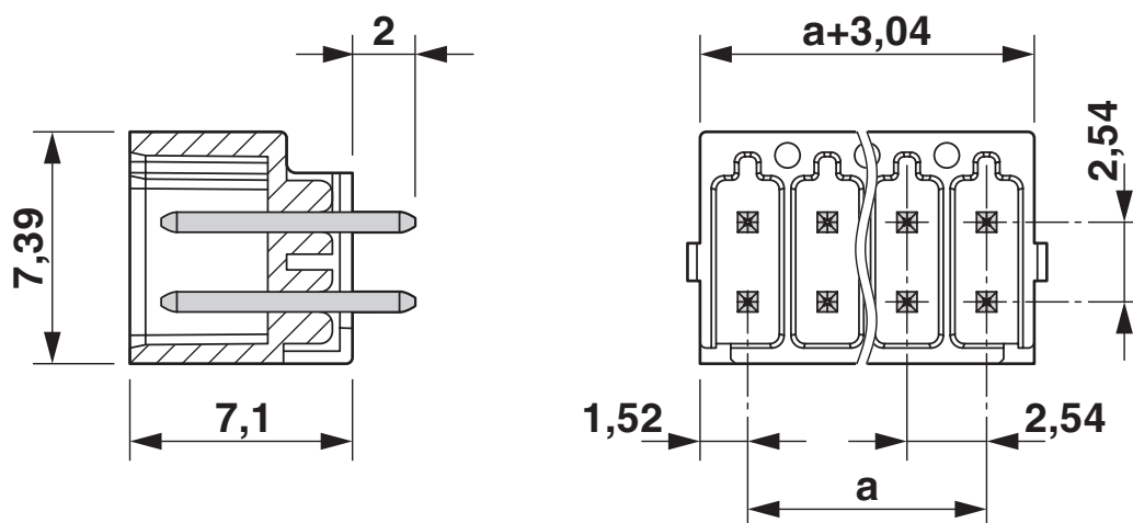
Rysunek wymiarowy
