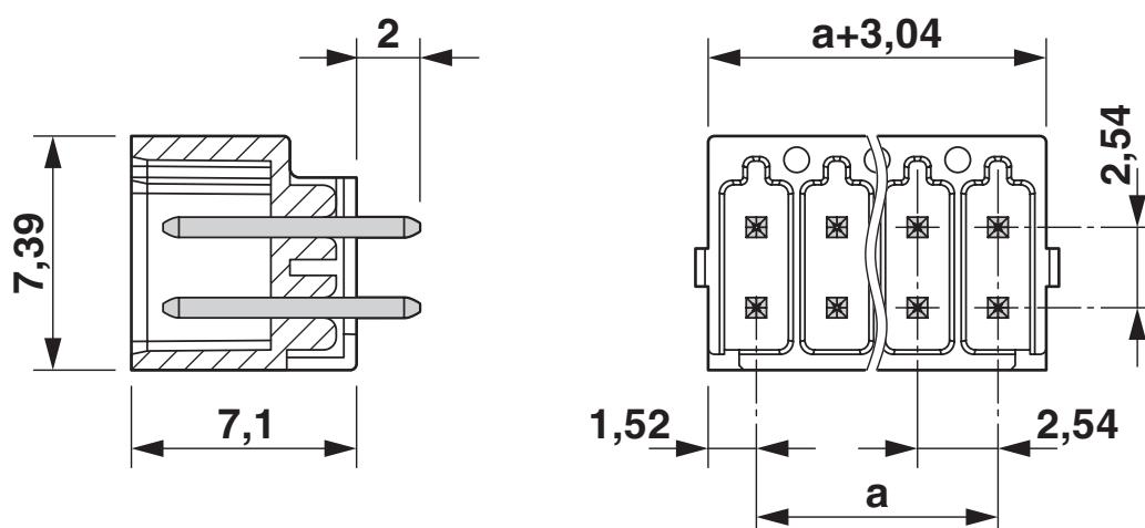
Rysunek wymiarowy
