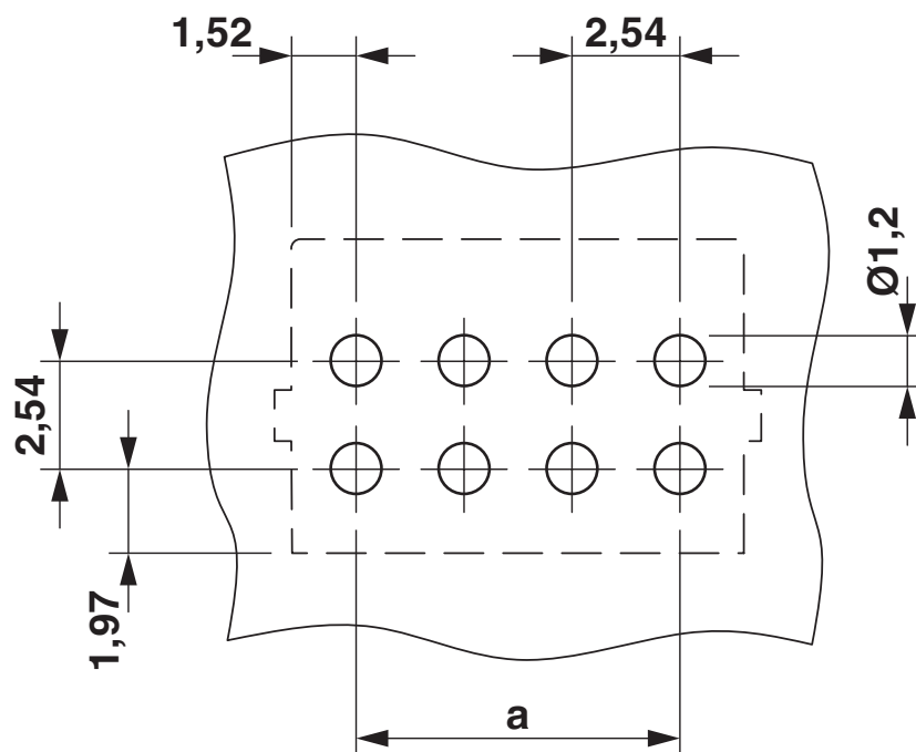
Otworowanie/geometria płytek lutowniczych
