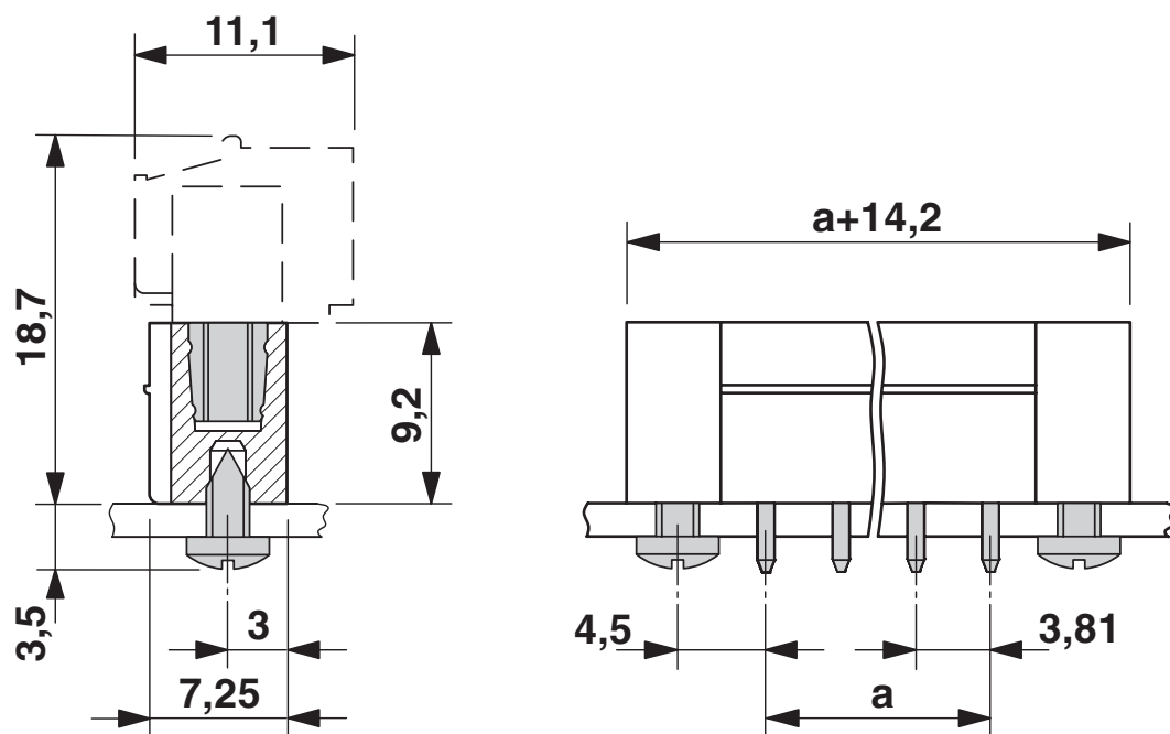
Rysunek wymiarowy
