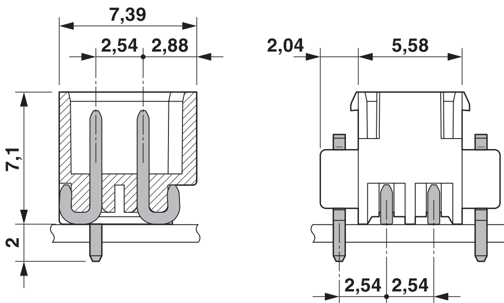
Rysunek wymiarowy
