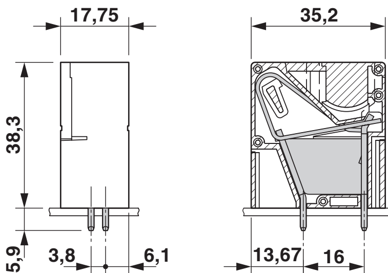
Rysunek wymiarowy
