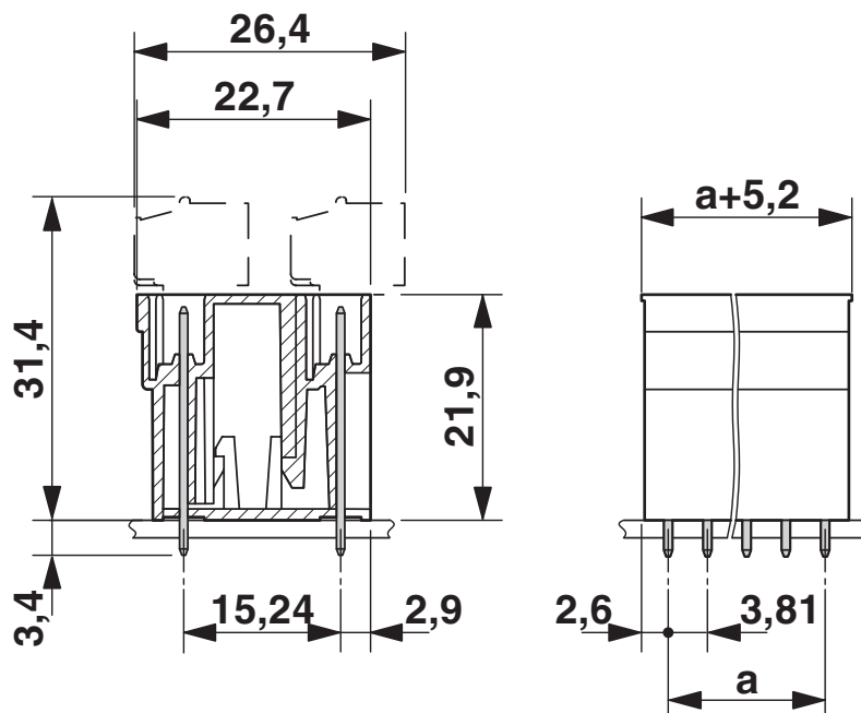
Rysunek wymiarowy
