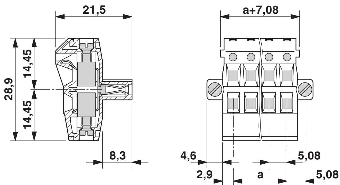
Rysunek wymiarowy
