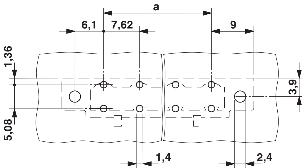
Otworowanie/geometria płytek lutowiczych
