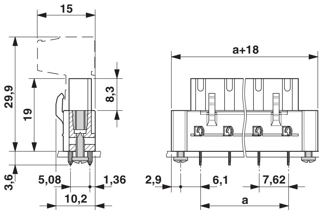
Rysunek wymiarowy
