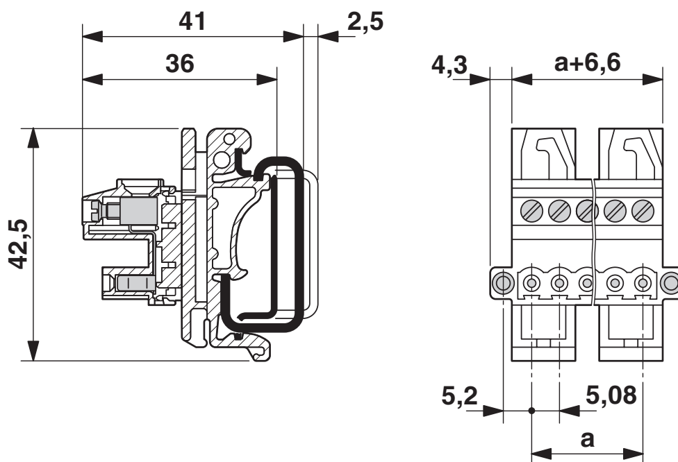
Rysunek wymiarowy
