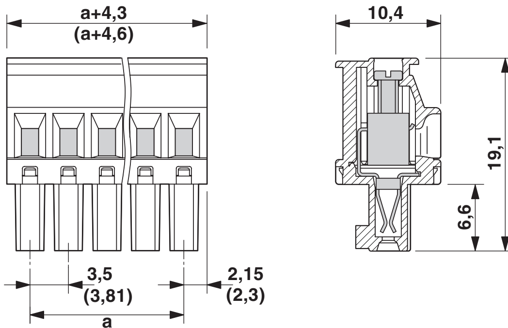
Rysunek wymiarowy
